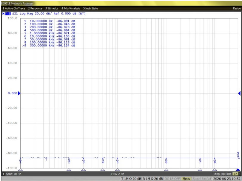
CCM 035300K 卡式宽带电流监测钳 s21 曲线
